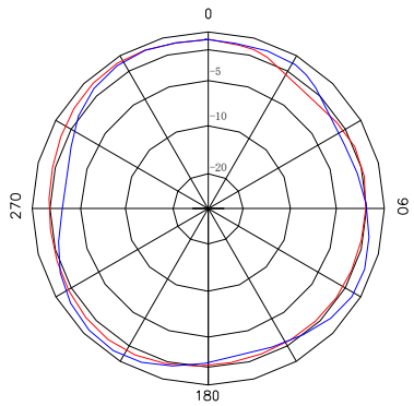
水平面方向图 (PCB板天线) Horizontal Pattern
