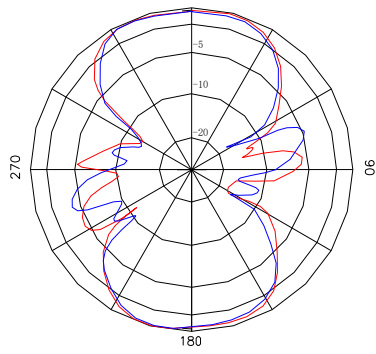
垂直面方向图 (PCB板天线) Vertical Pattern
